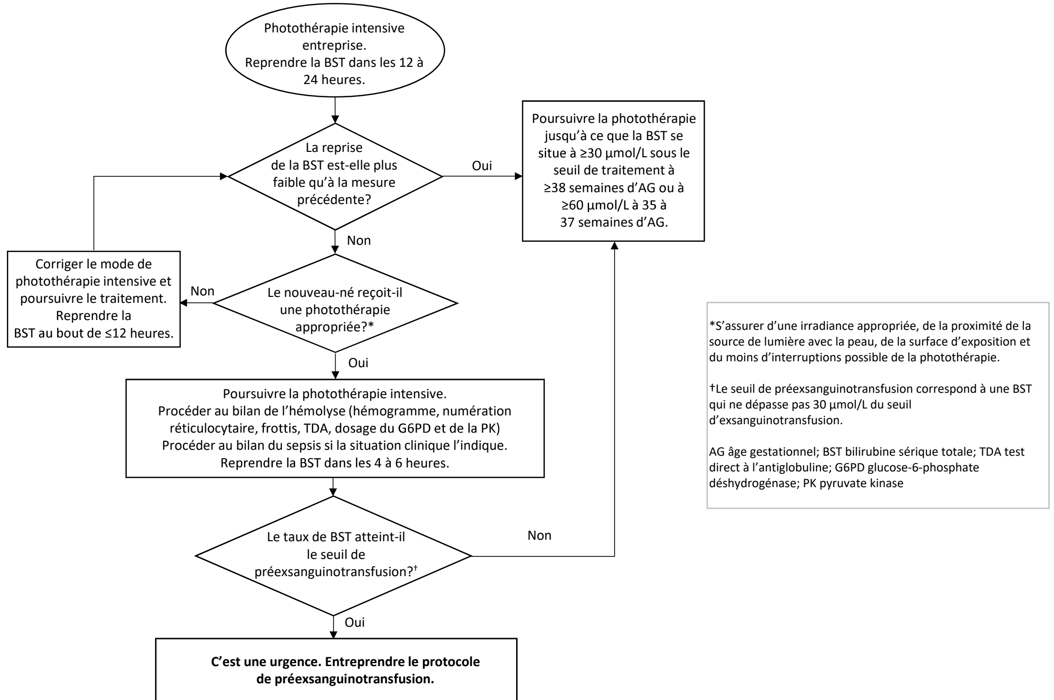
Figure 4. La surveillance des nouveau-nés pendant la photothérapie
