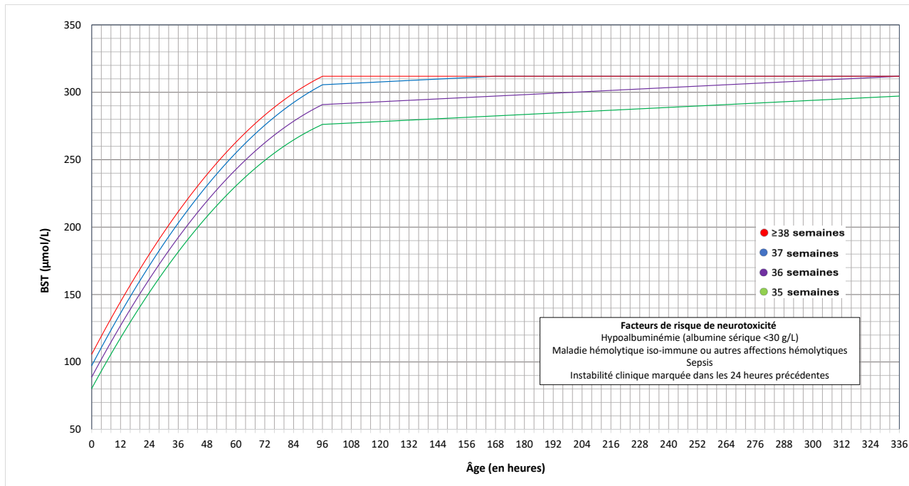
Figure 3. Les seuils de photothérapie des nouveau-nés présentant des facteurs de risque de neurotoxicité (données fournies par l'AAP; utilisation autorisée)
